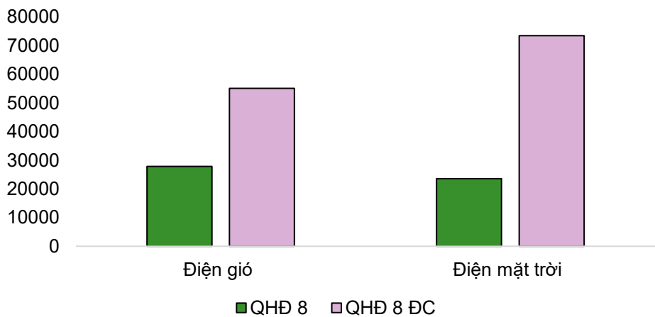
Tổng công suất nguồn theo QHĐ 8 ĐC tăng so với QHĐ 8
